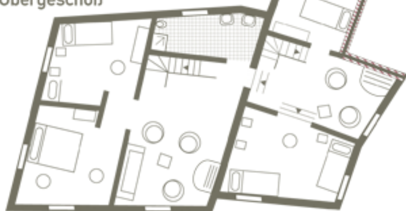
Obergeschoß
